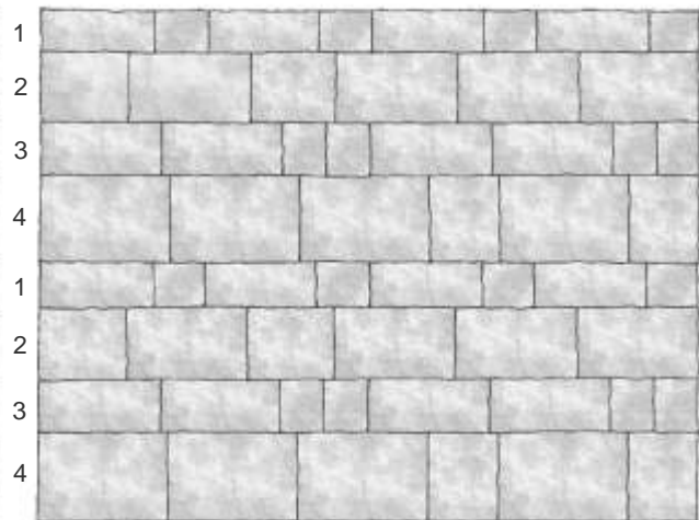
Pflasterbild nach Austausch der Wechselsteine
